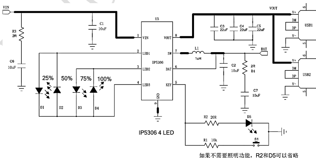
图 1 简化应用原理图(4 LED 指示电量)
