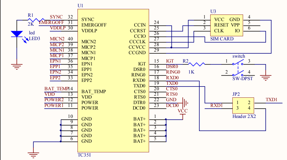
ZIF SIM
